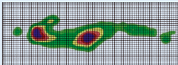
Bonellfederkernmatratze, 2,4 mm Federstahl, 7 x 24 Federn, Viergang: Auflagedruck bis zu 50 mmHG, Schlechte Druckverteilung
